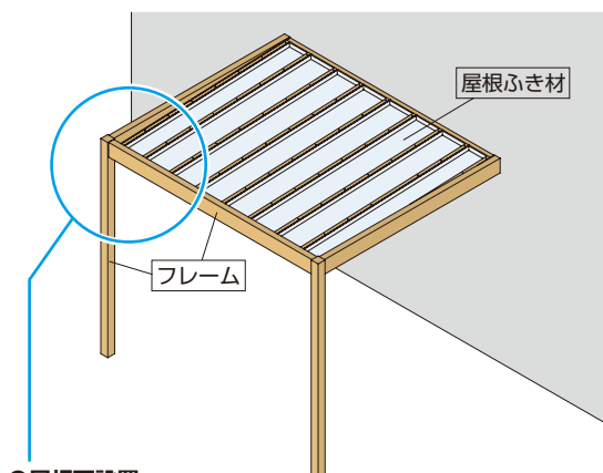
●屋根下設置 オプション:サンシェードカーテンⅡ ▶P.1634
