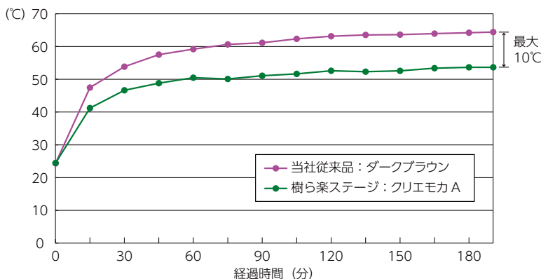
新旧製品の表面温度比較グラフ
