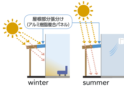
屋根部分張分け (アルミ樹脂複合パネル:厚さ3mm)
