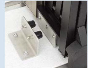
閉扉時の吊元枠ストップ機構。
