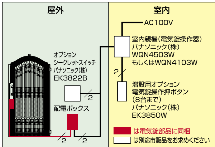
システム参考図(電気錠)
