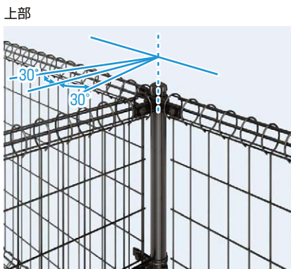
●T字角柱用部品(スチール) 水平方向に±30°の角度まで対応できます。
