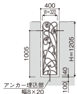
寸法図: 縮尺1/50 (単位mm)
