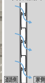
本体断面図
