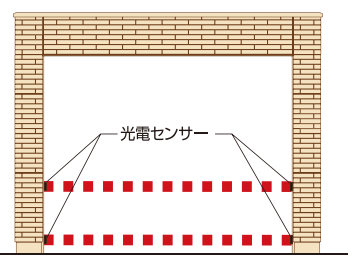
光電センサーは、高さ150mmと500mmの位置に設置されています。
