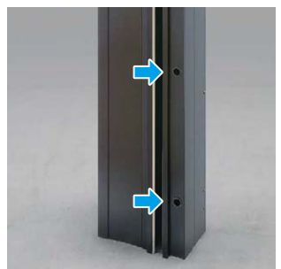
光電センサーは、高さ150mmと500mmの位置に設置されています。
