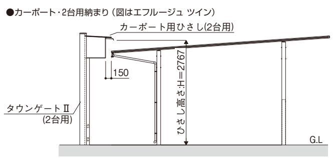
寸法図:縮尺1/100(単位mm)
