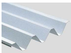
●スチール折板 (厚さt=0.6mm)
