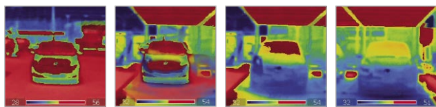
直射日光下 ポリカーボネート板 (グレー スモーク) 熱線遮断 ポリカーボネート板 (グレー スモーク) アルミ板
